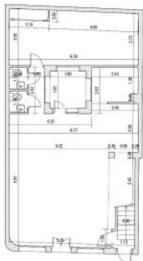
PLANTA BAJA
