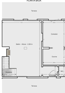
PLANTA BAJA
