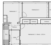
PRIMERA PLANTA
