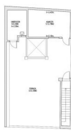
PLANTA CUBIERTA
