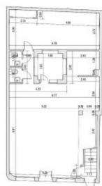
PLANTA BAJA
